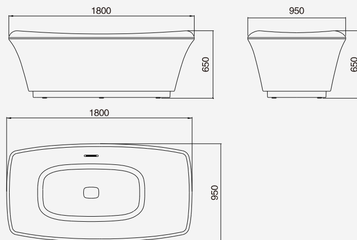
产品尺寸图
