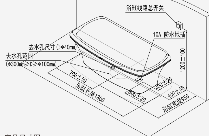
产品尺寸图
